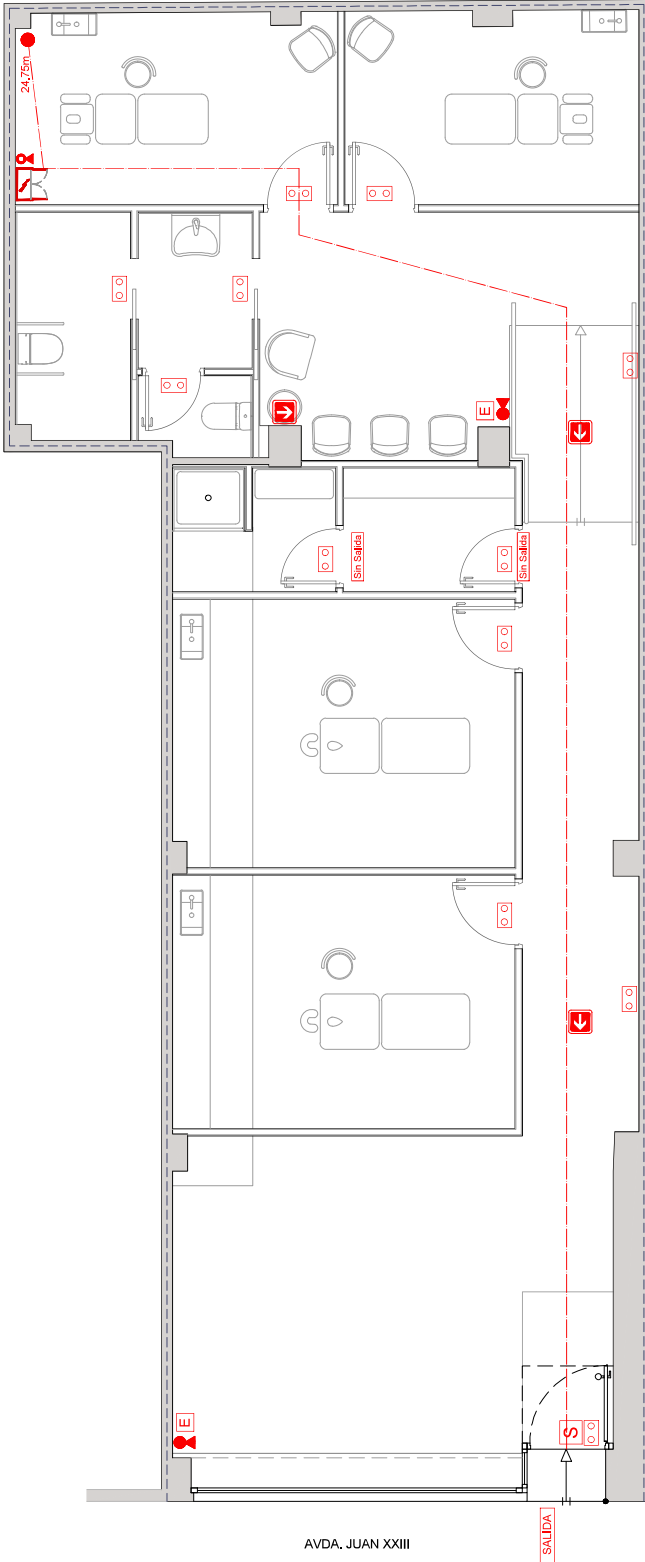
PLANO PROTECCIÓN CONTRA INCENDIOS
