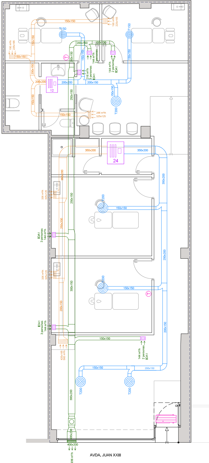
PLANO VENTILACIÓN Y CLIMATIZACIÓN ESCALA 1:50
