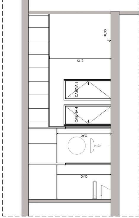
SECCIÓN B-B' PLANTA BAJA ESTADO ACTUAL ESCALA 1:50
